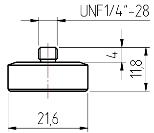
Artikel.-Nr.30000882 Haftmagnet UNF1/4"-28
