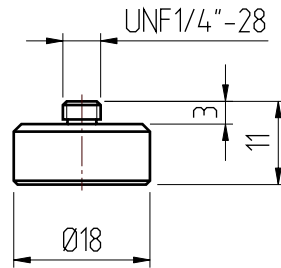
Artikel.-Nr.30000880 Haftmagnet UNF1/4"-28 kleines Magnetsystem (Ø10)
