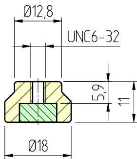
Artikel.-Nr.30000920 Haftmagnet UNC6-32 (innen) kleines Magnetsystem (Ø10)
