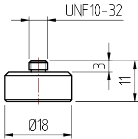
Artikel.-Nr.30000900 Haftmagnet UNF10-32 kleines Magnetsystem (Ø10)
