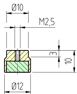
Artikel.-Nr.300009xx Haftmagnet M2,5 (innen)
