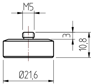
Artikel.-Nr.30000840 008 Haftmagnet M5
