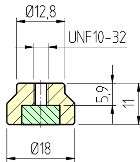
Artikel.-Nr.30000940 Haftmagnet UNF10-32 (innen) kleines Magnetsystem (Ø10)
