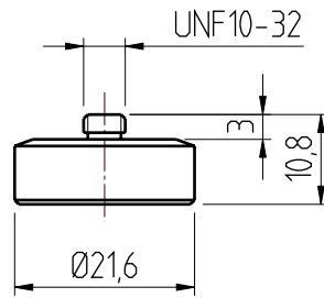
Artikel.-Nr.30000860 008 Haftmagnet UNF10-32
